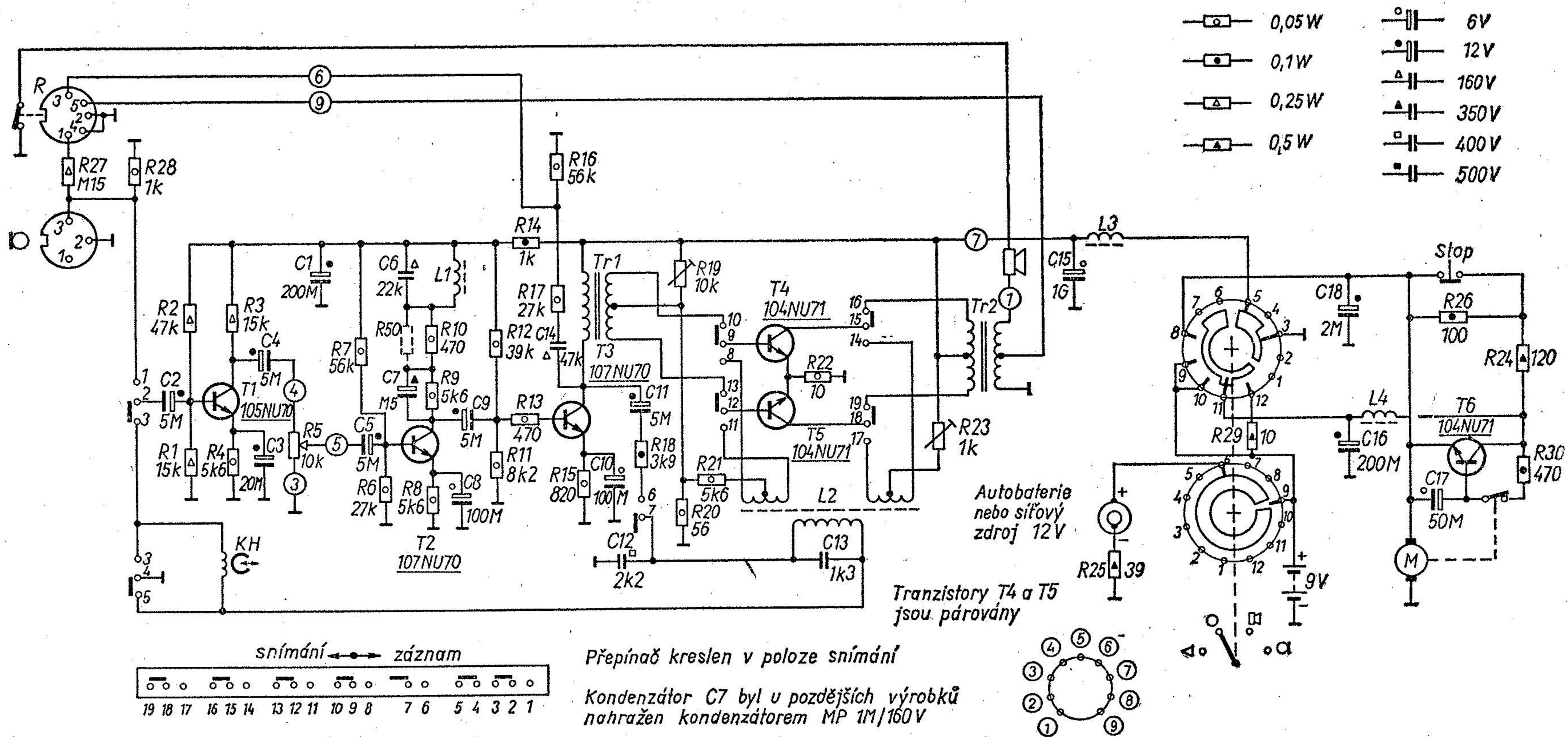
Obr. 132. Zapojení magnetofonu TESLA START ANP 402
