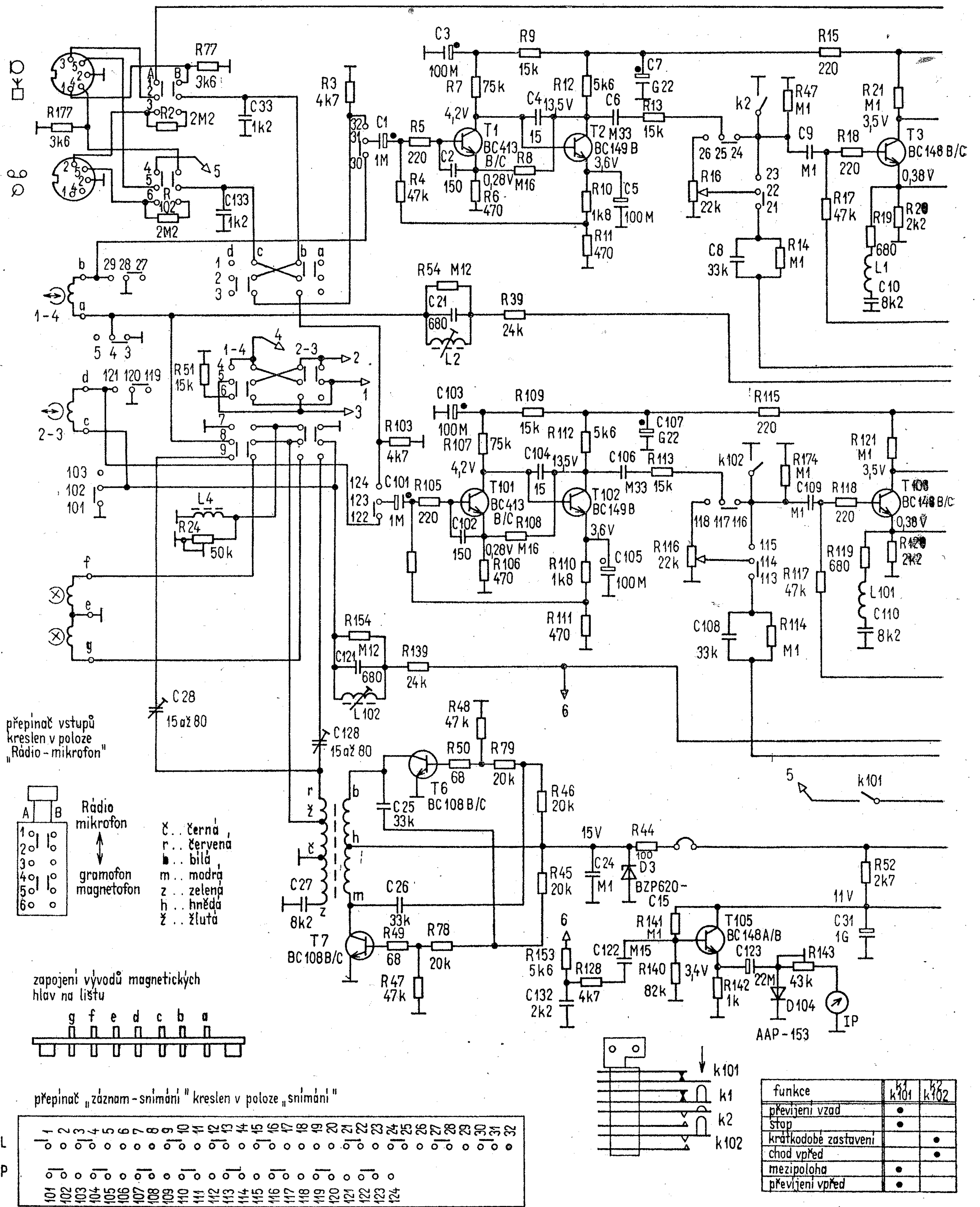
Zapojení magnetofonu M 1417 S
