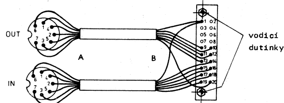
Zapojení kabelu (pohled ze strany pájecích bodů)
