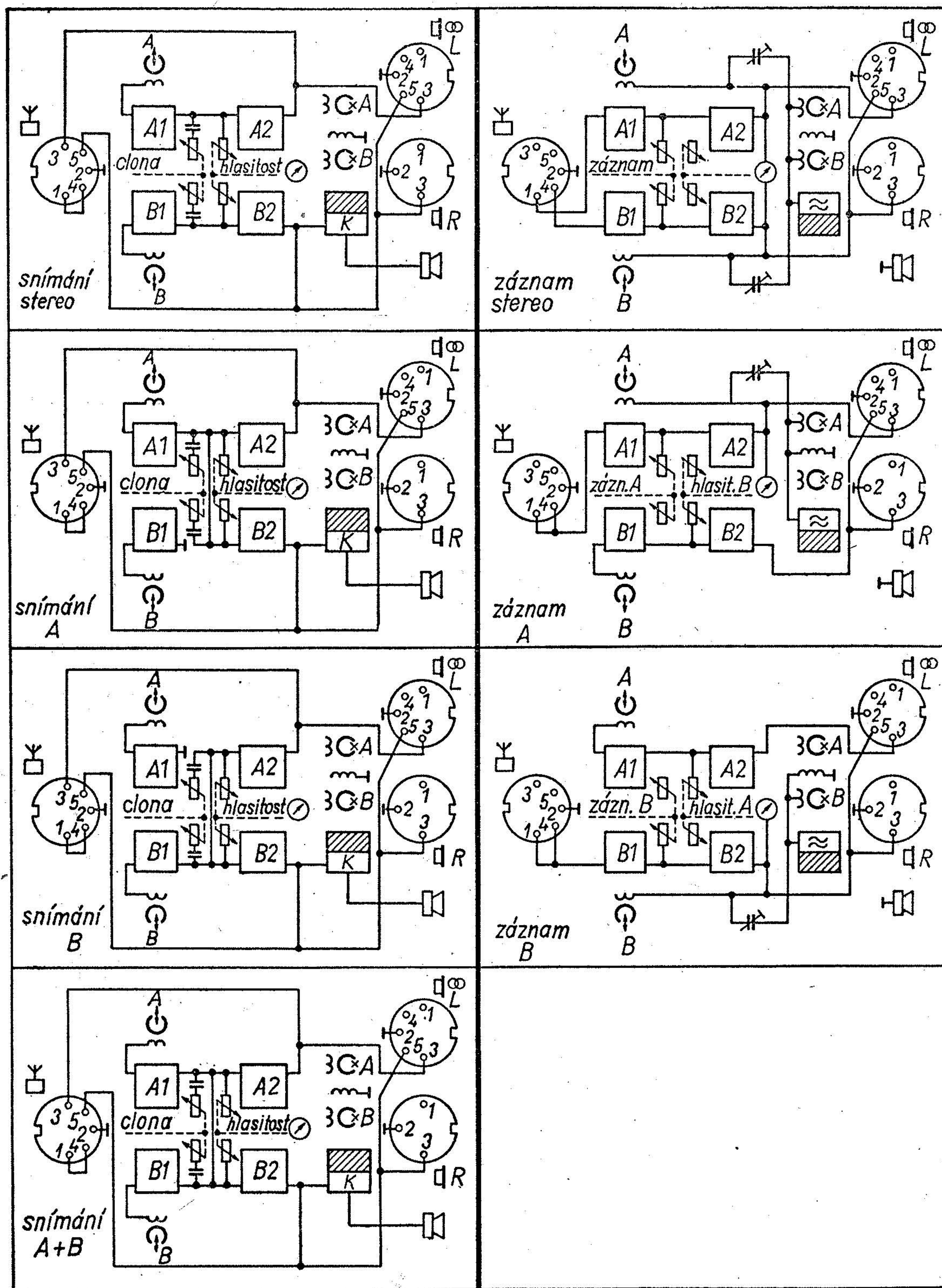
Obr. 112. Blokova schémata magnetofonu TESLA B 46
